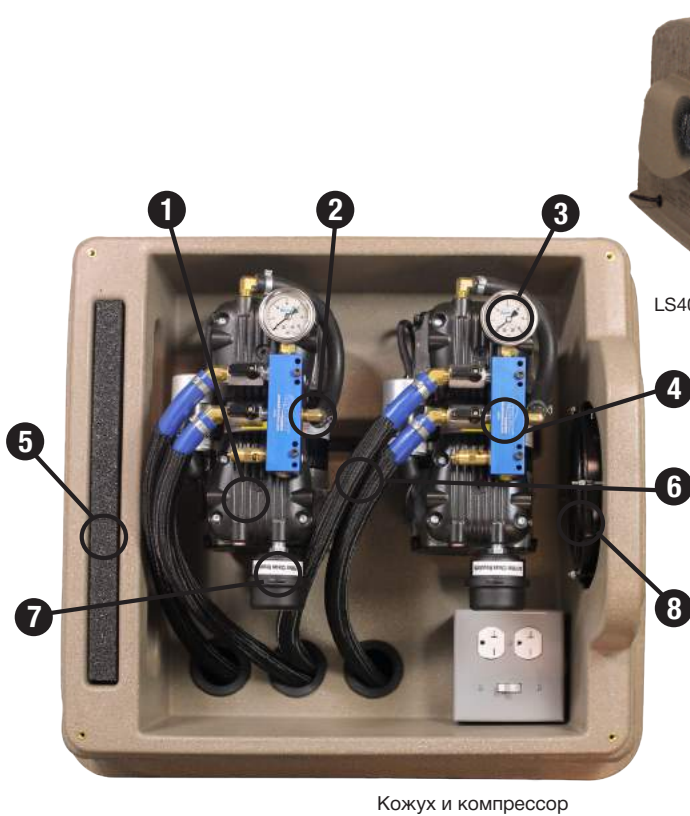
Кожух и компрессор
